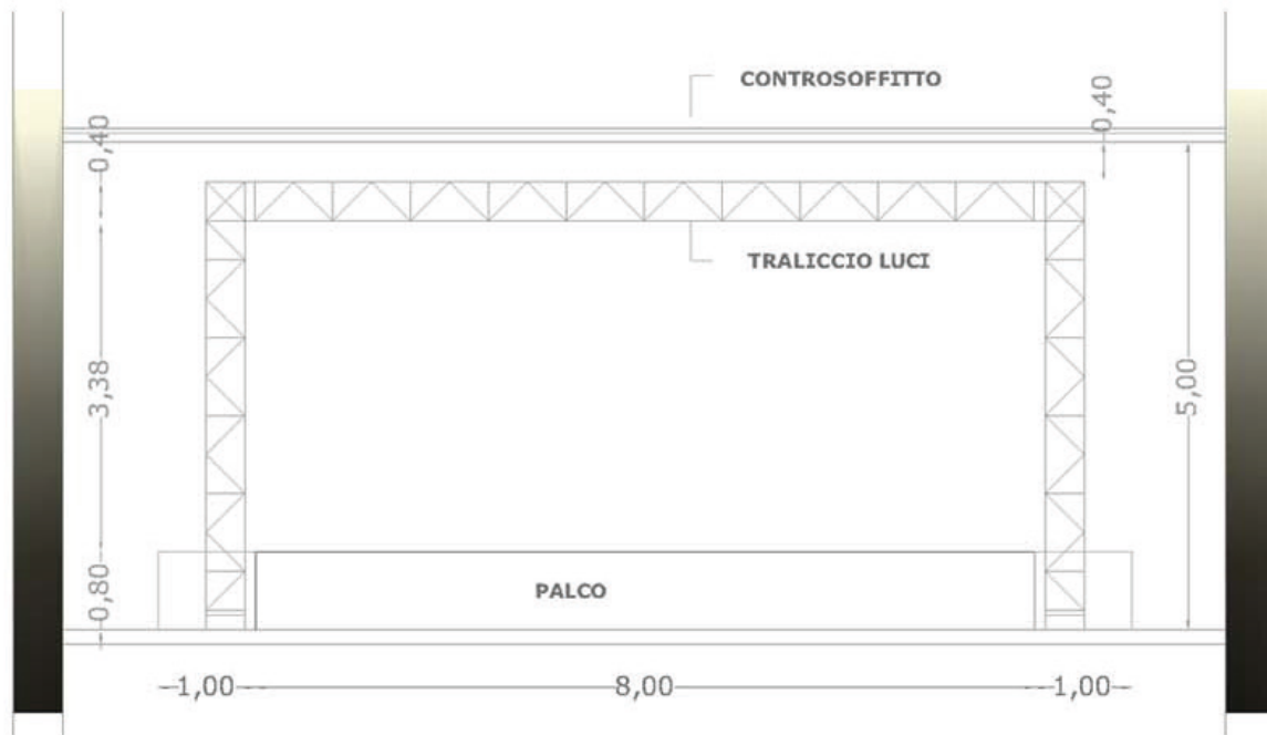
SEZIONE TRASVERSALE
